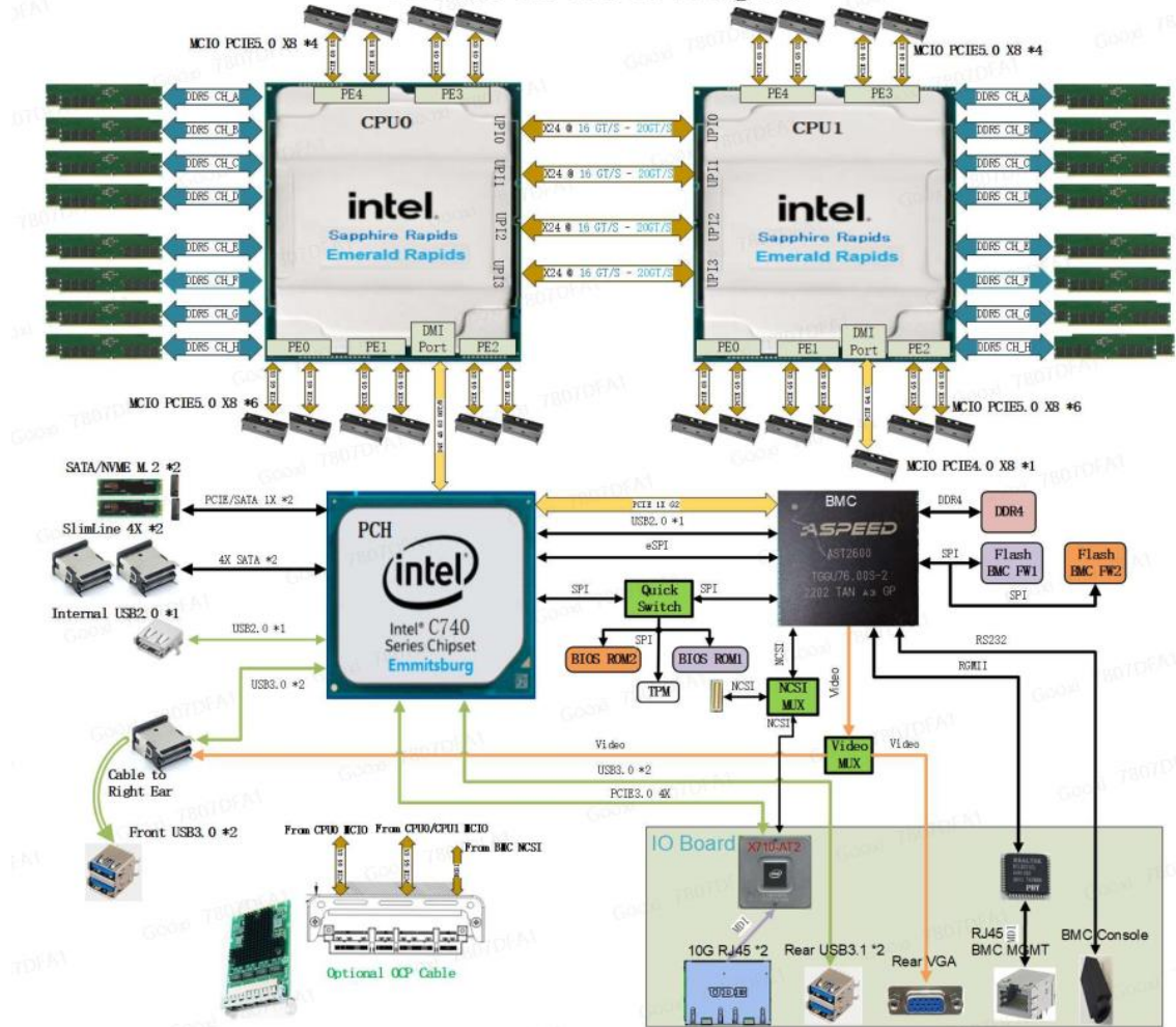
主板逻辑框图 1-2
