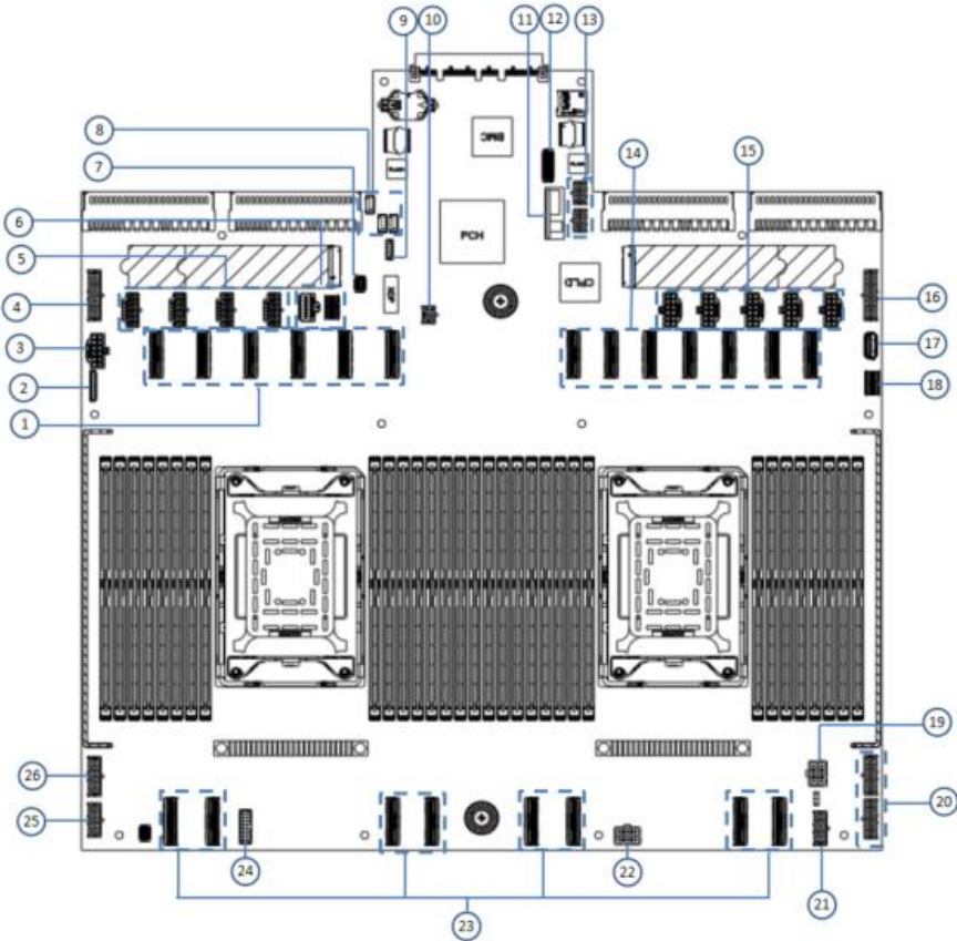
主板图 2-14
